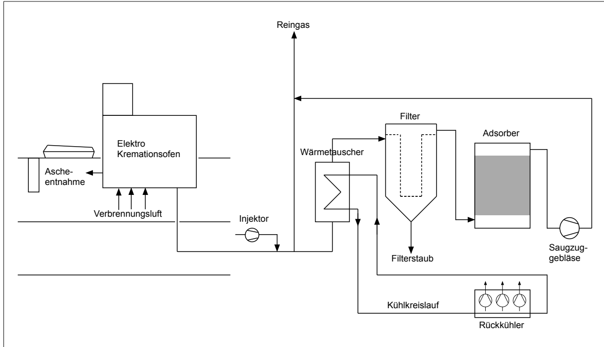
Abbildung 8: Vereinfachtes Verfahrenflussbild bestehende Ofenlinie
